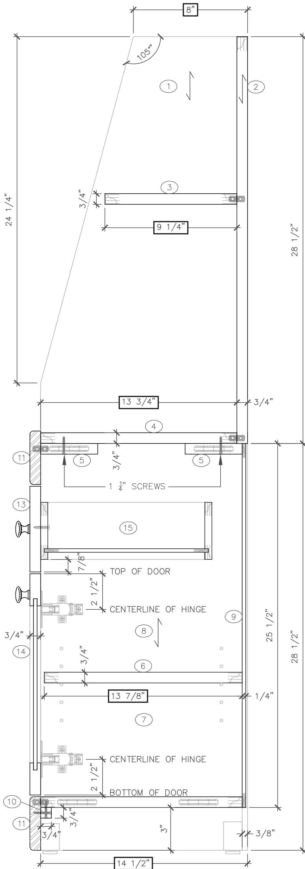
C SECTION SCALE: 3"=1'-0"
