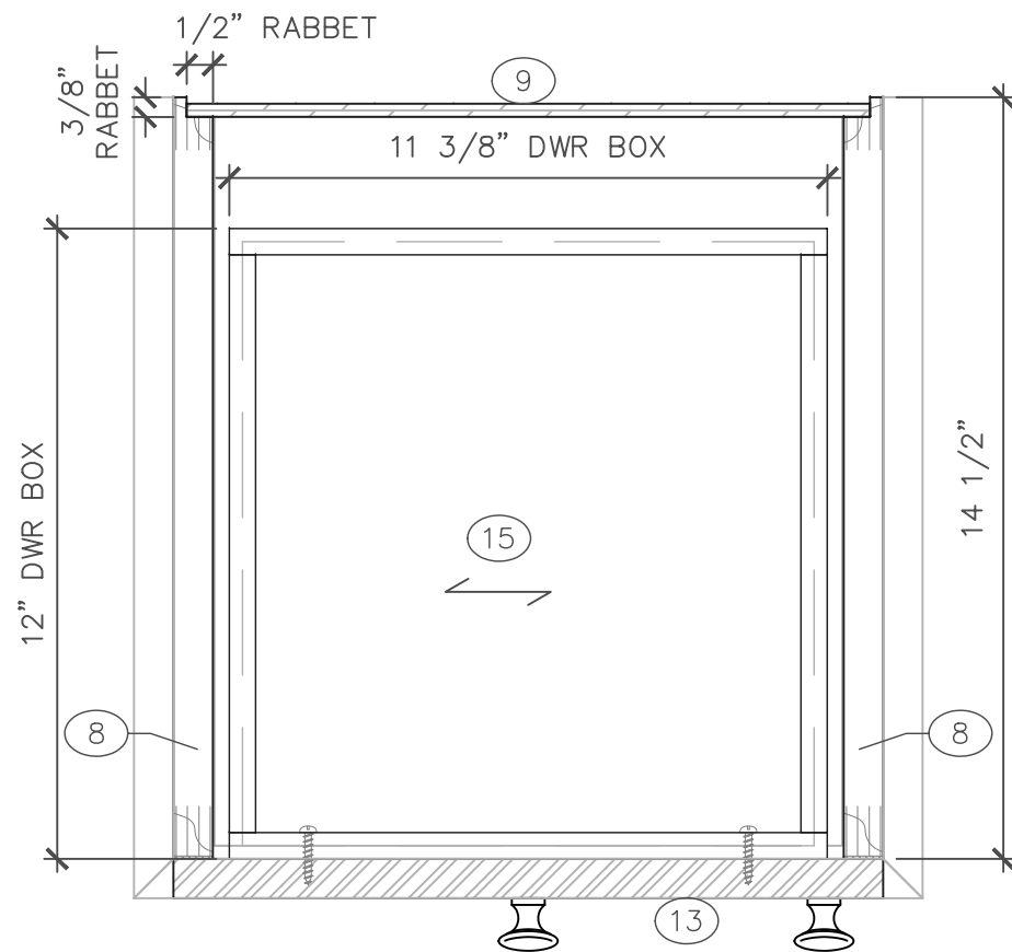
H SECTION SCALE: 1-1/2"=1'-0"
