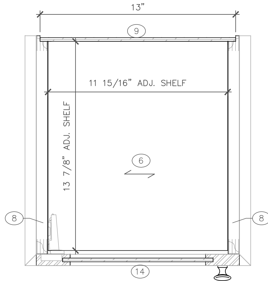
I SECTION SCALE: 1-1/2"=1'-0"
