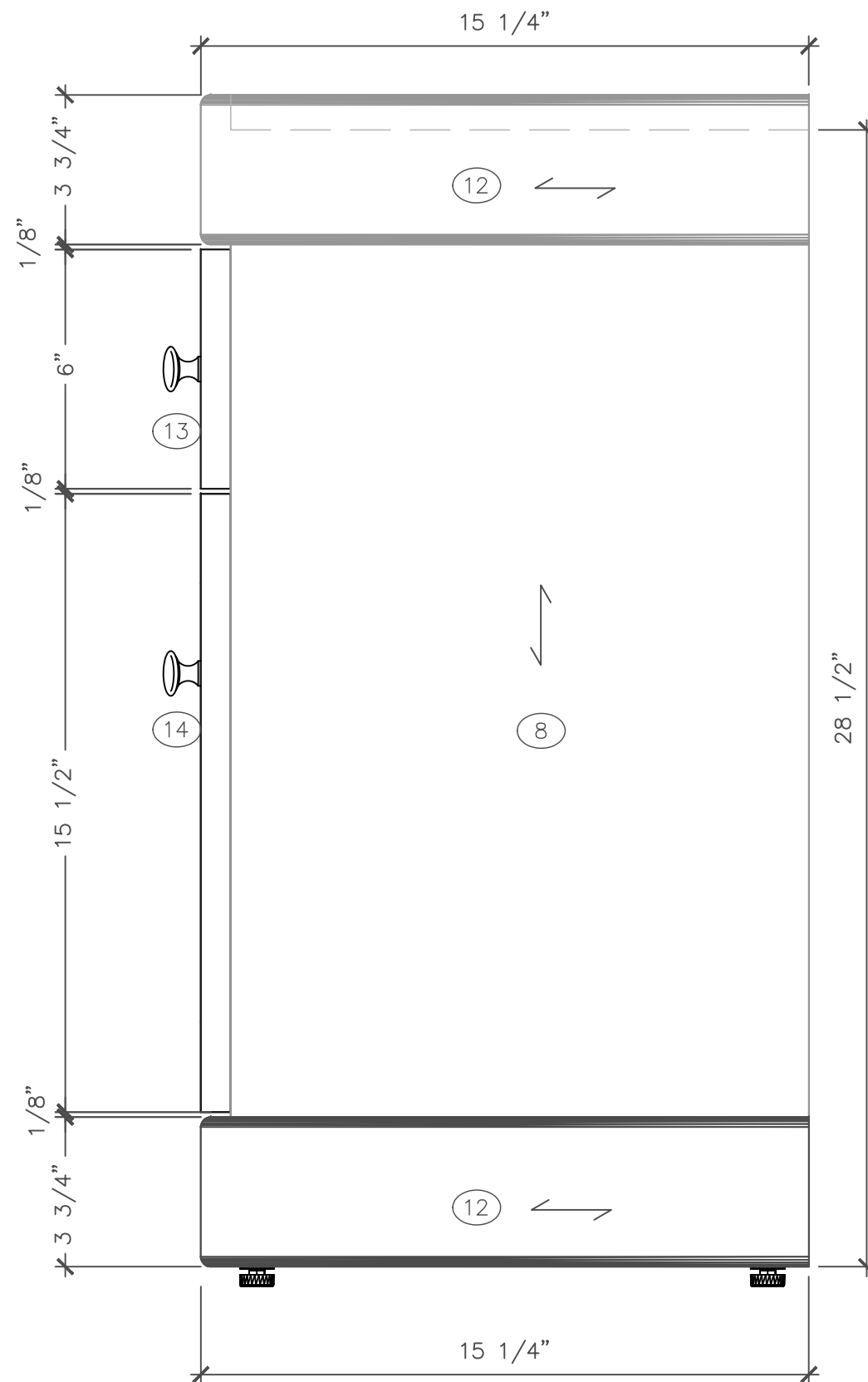
E CAB ELEVATION SCALE: 3"=1'-0"
