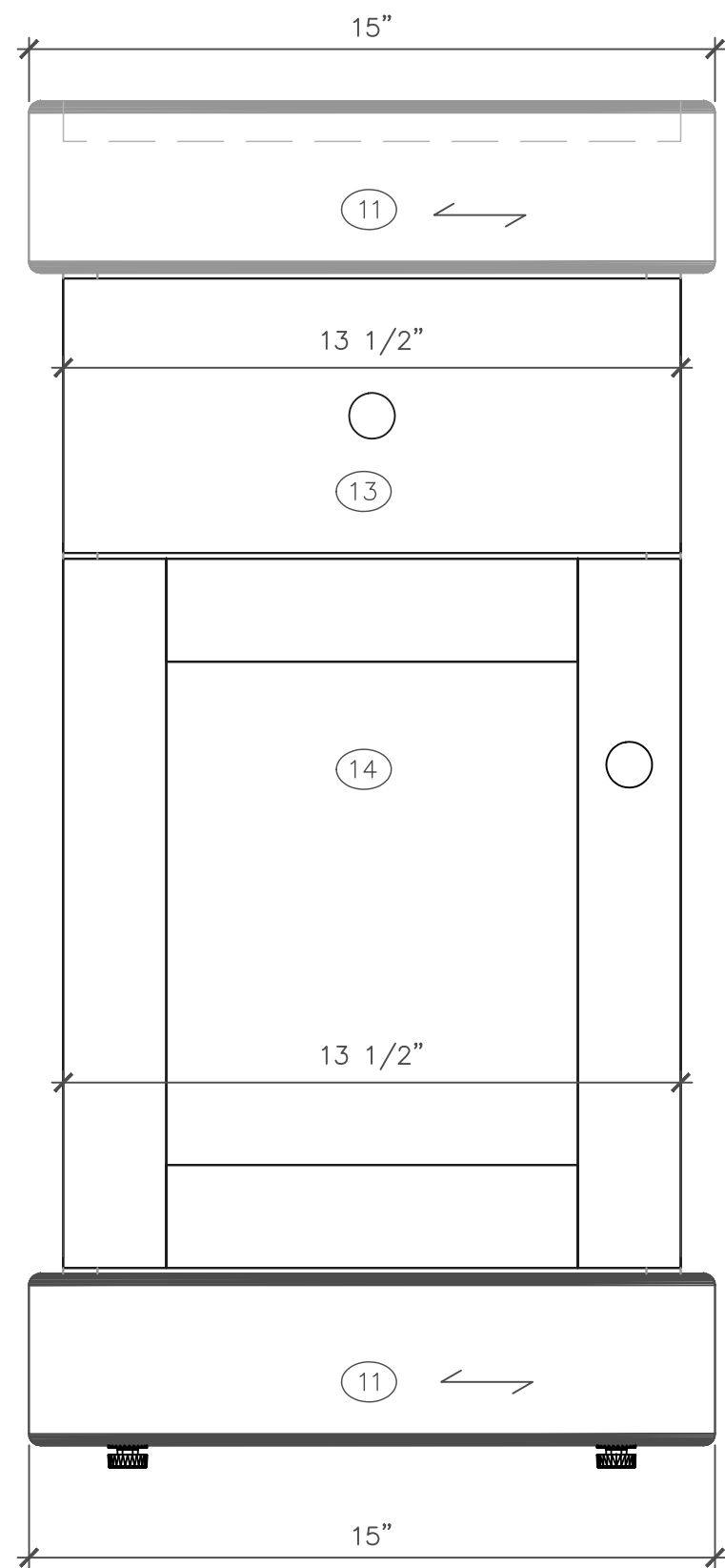
D CAB ELEVATION SCALE: 3"=1'-0"
